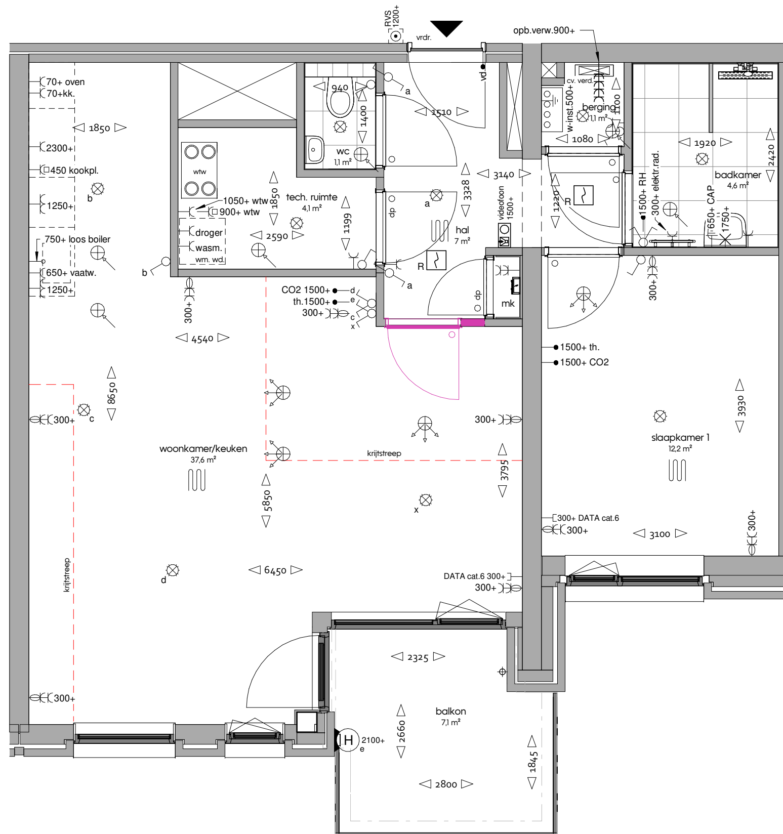
Baltimore, type B, optie B1-201 slaapkamer 2 samenvoegen met woonkamer
